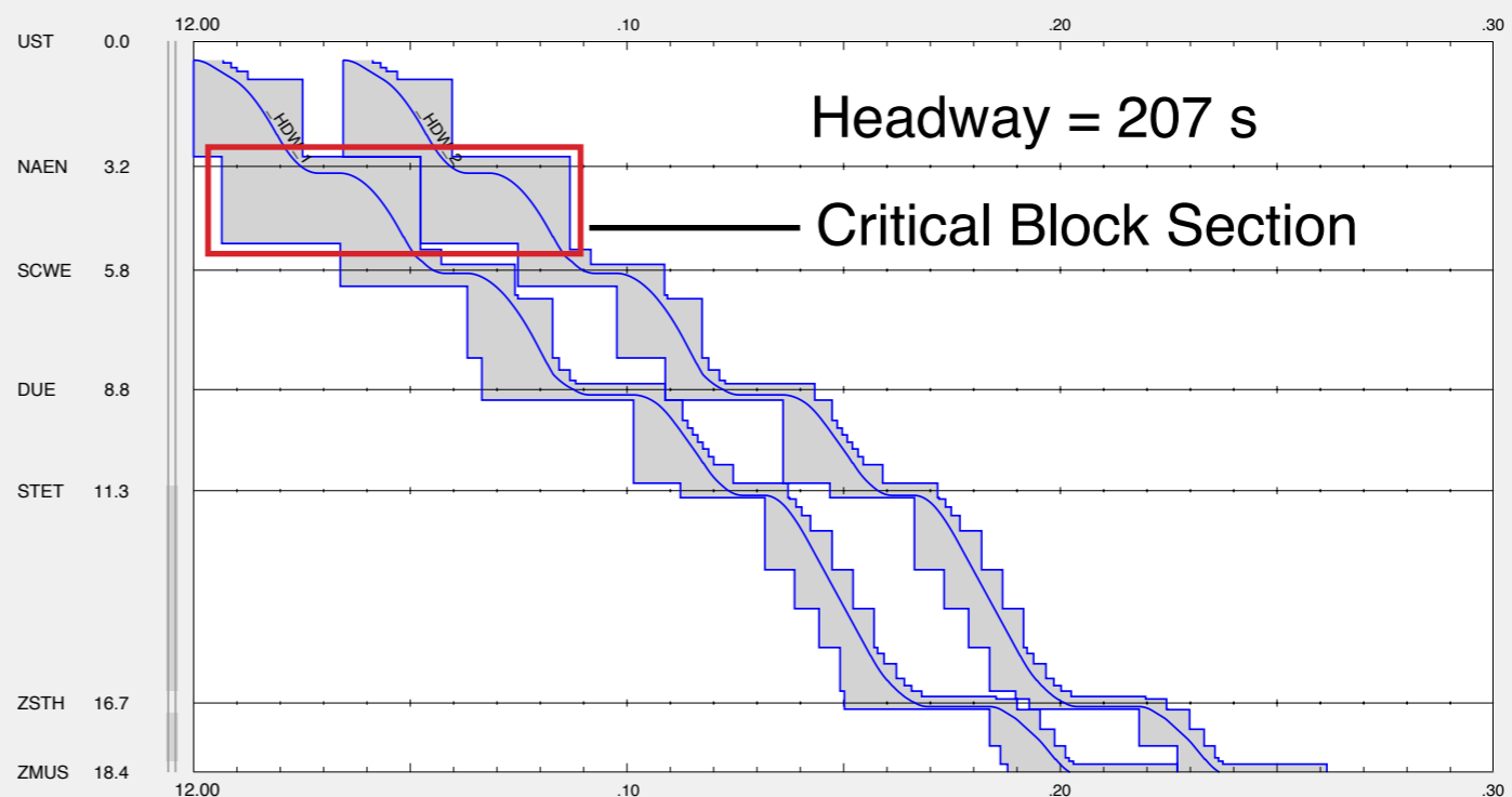
UST-ZMUS: Headway Calculation Uster - Zurich
